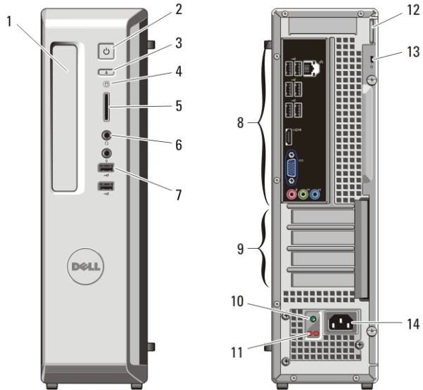
איור 2. מבט מלפנים ומאחור של Slim Tower
