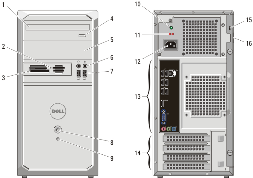
איור 1. מבט מלפנים ומאחור של Mini Tower
