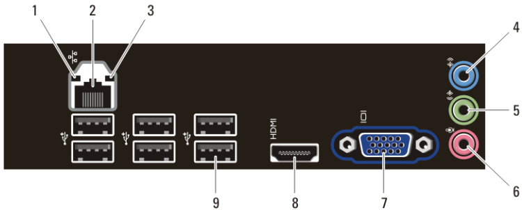
איור 3. מבט על הלוח האחורי של מחשב Mini Tower ומחשב Slim Tower
